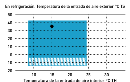
Rango de temperatura para bodega de vino.
