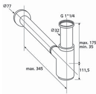
919.639.6 GENESIS lavabo latón.
