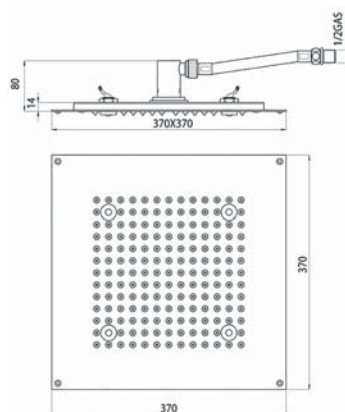
H37452 DREAM OKI. Consumo mínimo 14 l/min.
