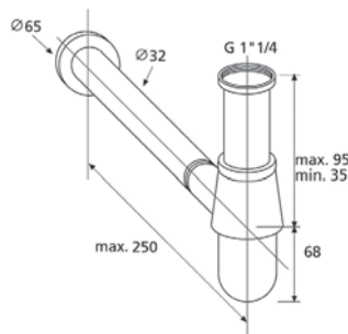
19.225.5 BOTELLA lavabo latón.
