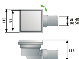
2565.521.8 Sumidero horizontal KUALA LUMPUR 120x120 mm. Sifón extraíble.
