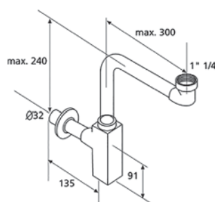
811.136.5 QUASAR-EXEL lavabo latón.
