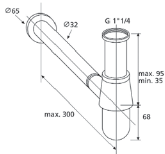
19.235.5 BOTELLA lavabo latón.
