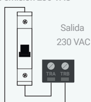
Bobina de emisión 230 VAC
