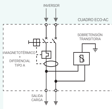
Esquema tipo ECO-AC-1NT15
