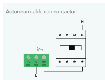
Esquema conexionado V3P3.0
