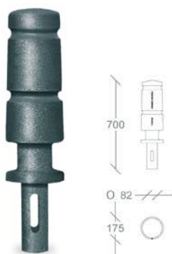
▲ CIBELES Mod. C-602
