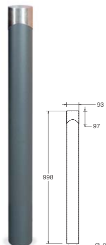
DUNA Mod. C-525
