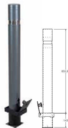
▲ ECO Mod. C-43D-ECO
