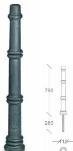
▲ MADRID Mod. C-509
