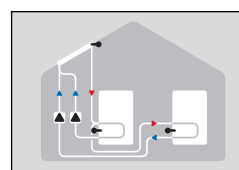
Solar con dos almacenamientos y dos bombas
