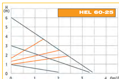
BOMBA HEL 60/25
