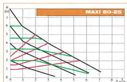
BOMBA MAXI 80/25
