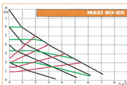
BOMBA MAXI 80/25
