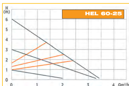
BOMBA HEL 60/25
